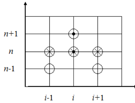
4.1 pav. (4.2) skirtuminę schemą atitinkantis šablonas. \circ – išvestinės \frac{\partial}{\partial t} \left( \frac{\partial^2 u}{\partial x^2} \right) aproksimavimo taškai.
