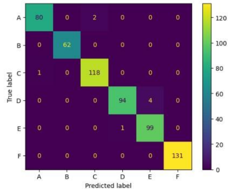
(d) convmixer_768_32
