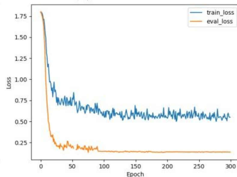
(d) convmixer_768_32
